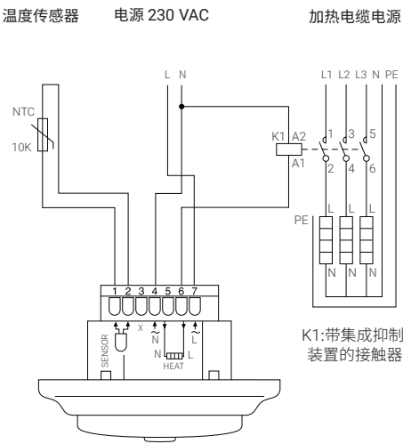
通过接触器连接, 比如3个加热回路
